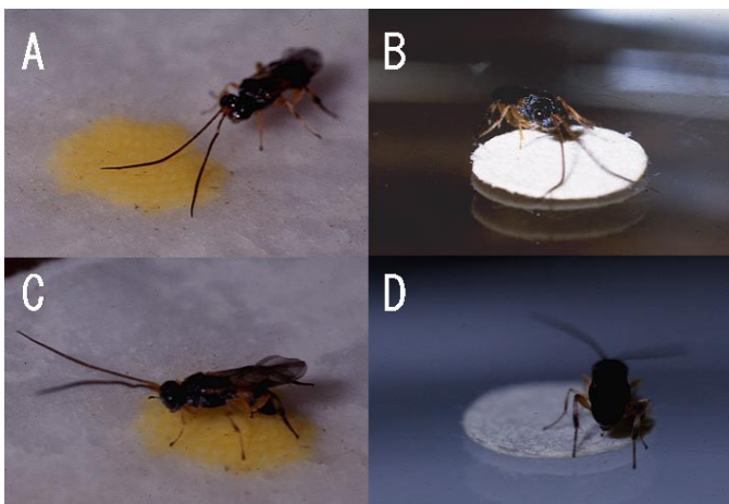
写真2. 寄主卵塊に対する触角での反応 (A) や産卵管挿入行動 (C) は、卵塊抽出物を処理したろ紙に対しても見られる (B, D)
