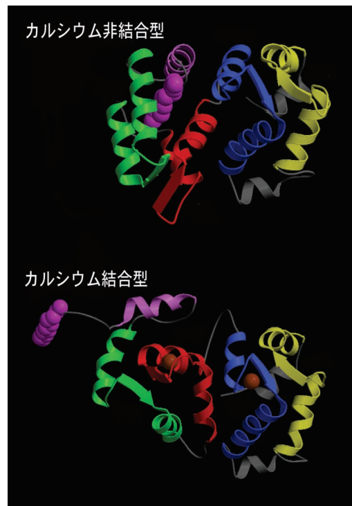
図2. 蛋白質の構造変化の様子。カルシウム結合蛋白質リカバリンは、カルシウム(図ではオレンジ)を結合すると、それまで自分の中にしまっておいた脂肪酸(図では紫)を飛び出させ、細胞膜に結合するが、NMR解析でその様子を見事に捉えることが出来た。
